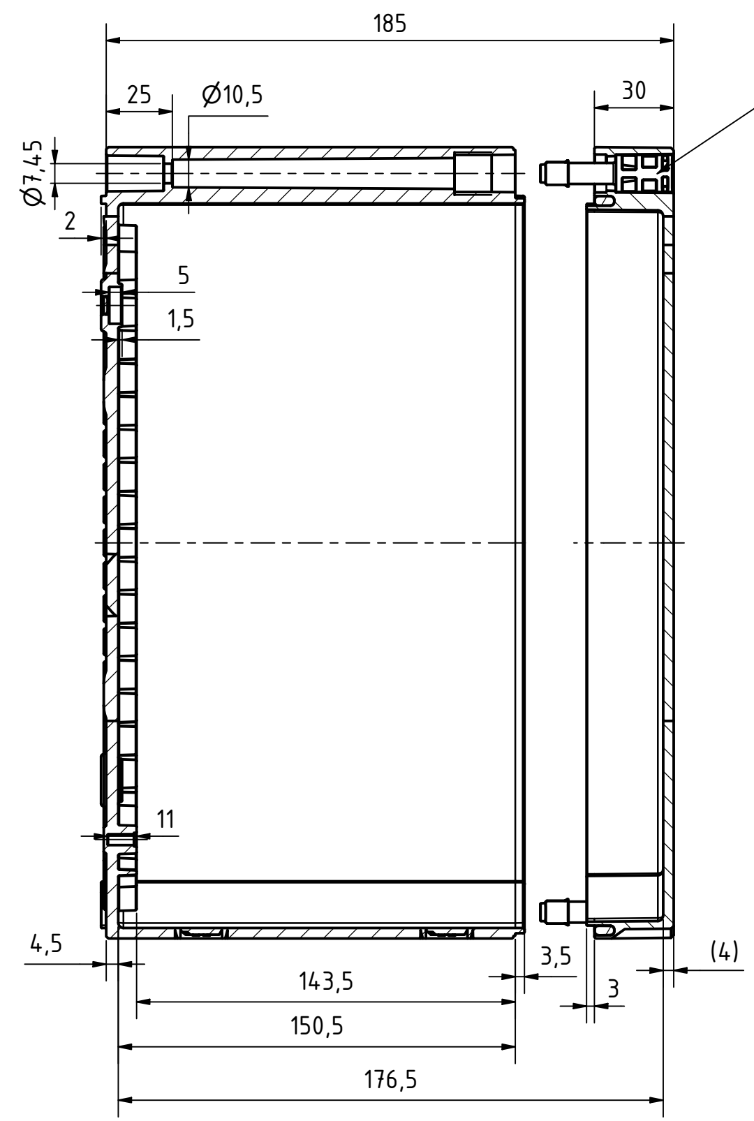
A-A ( 1 : 2 )
