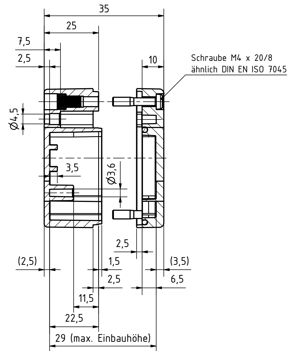
A-A ( 1 : 1 )
