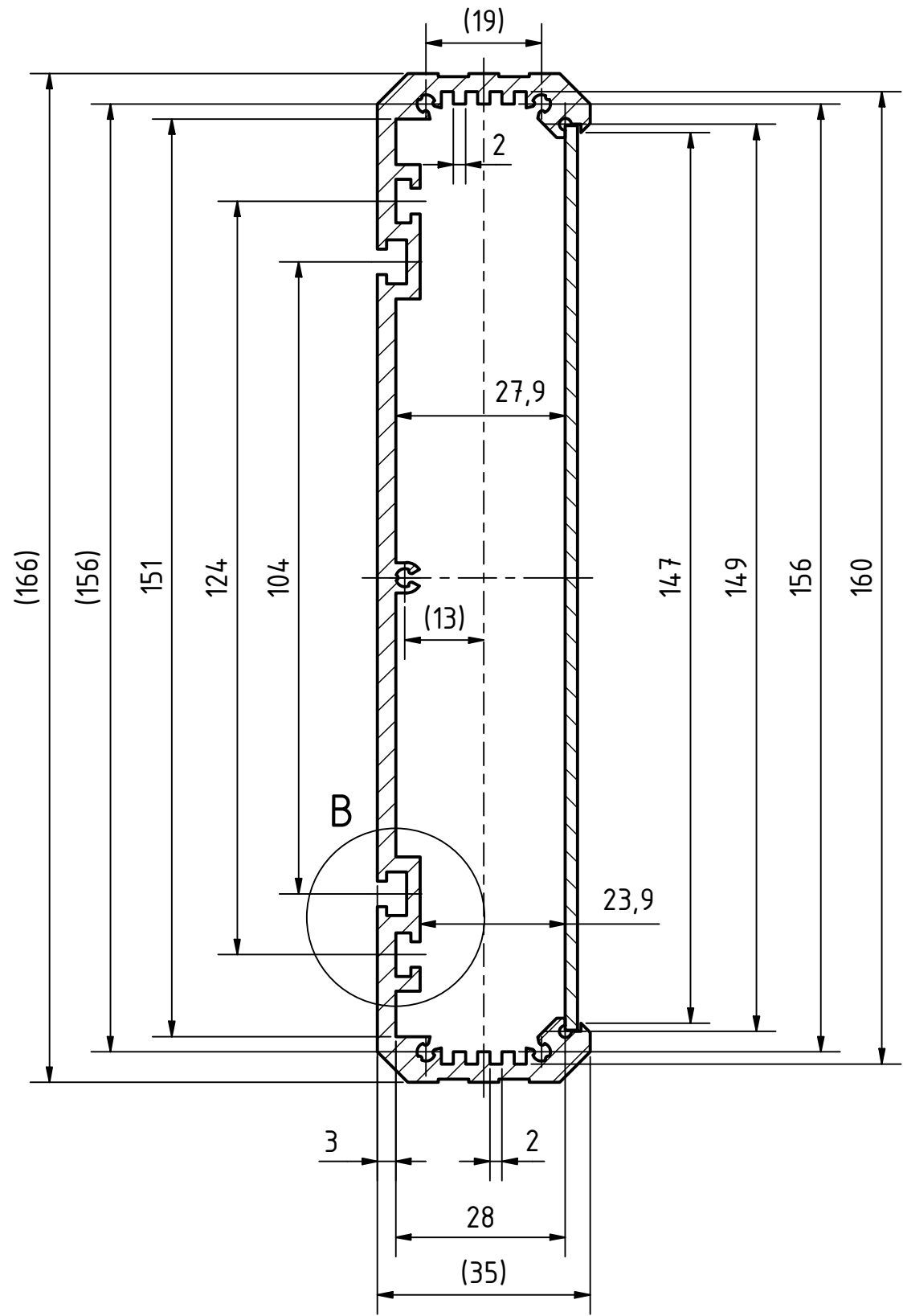
A-A Querschnitt Profil und Frontplatte
