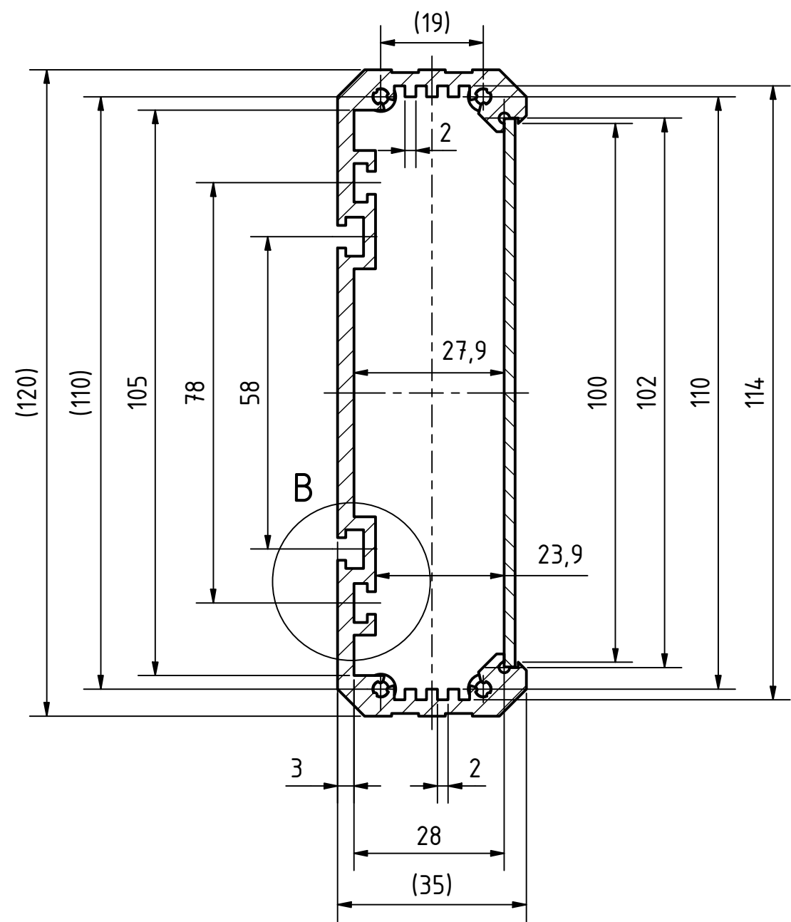
A-A Querschnitt Profil und Frontplatte
