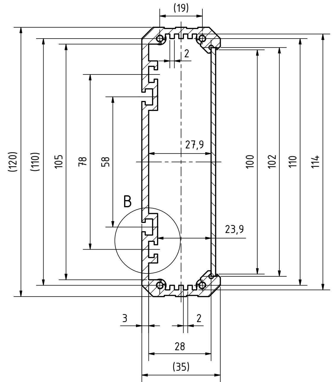
A-A Querschnitt Profil und Frontplatte
