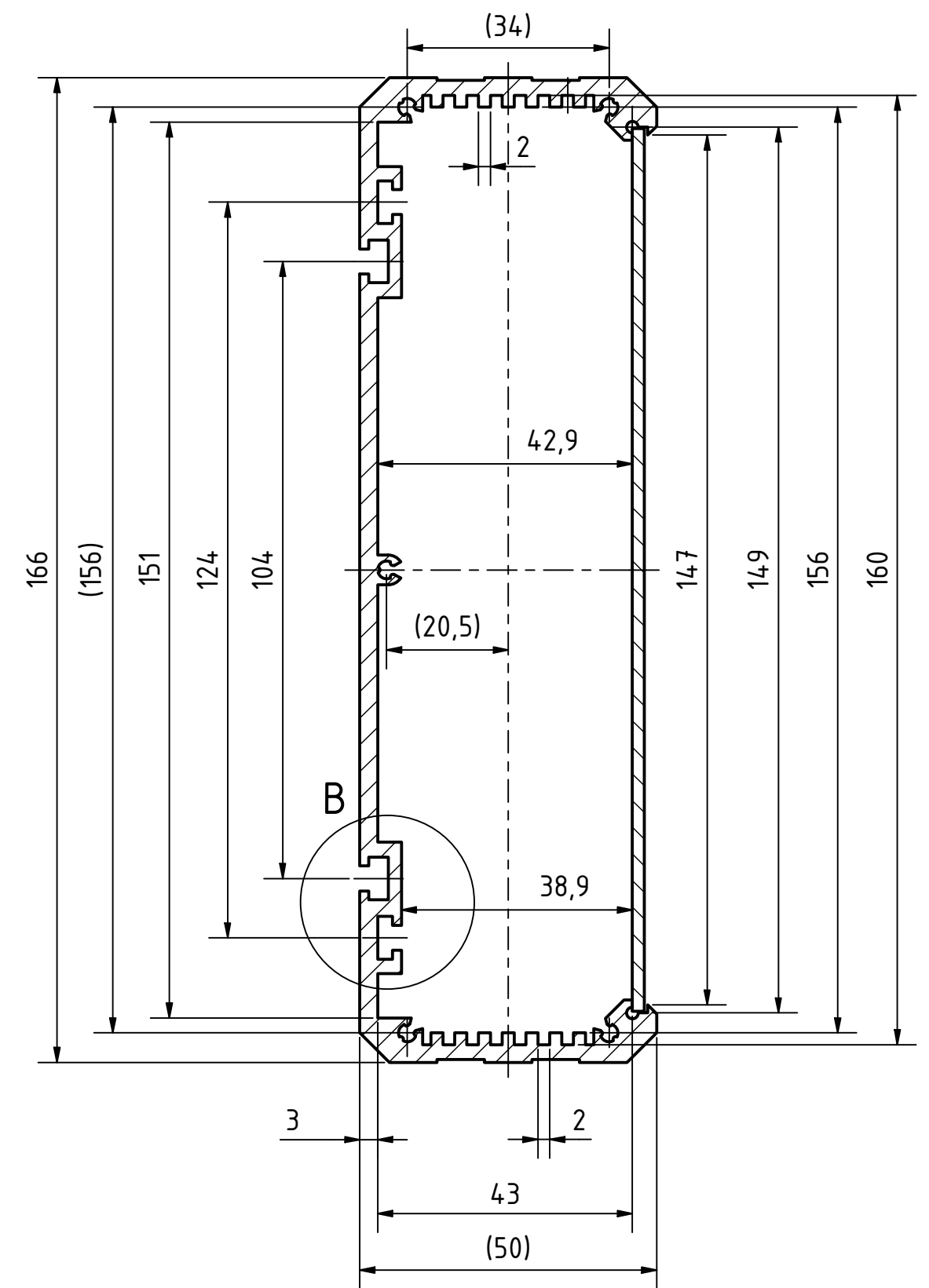
A-A Querschnitt Profil und Frontplatte
